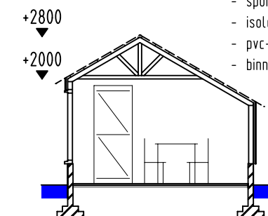
Doorsnede
