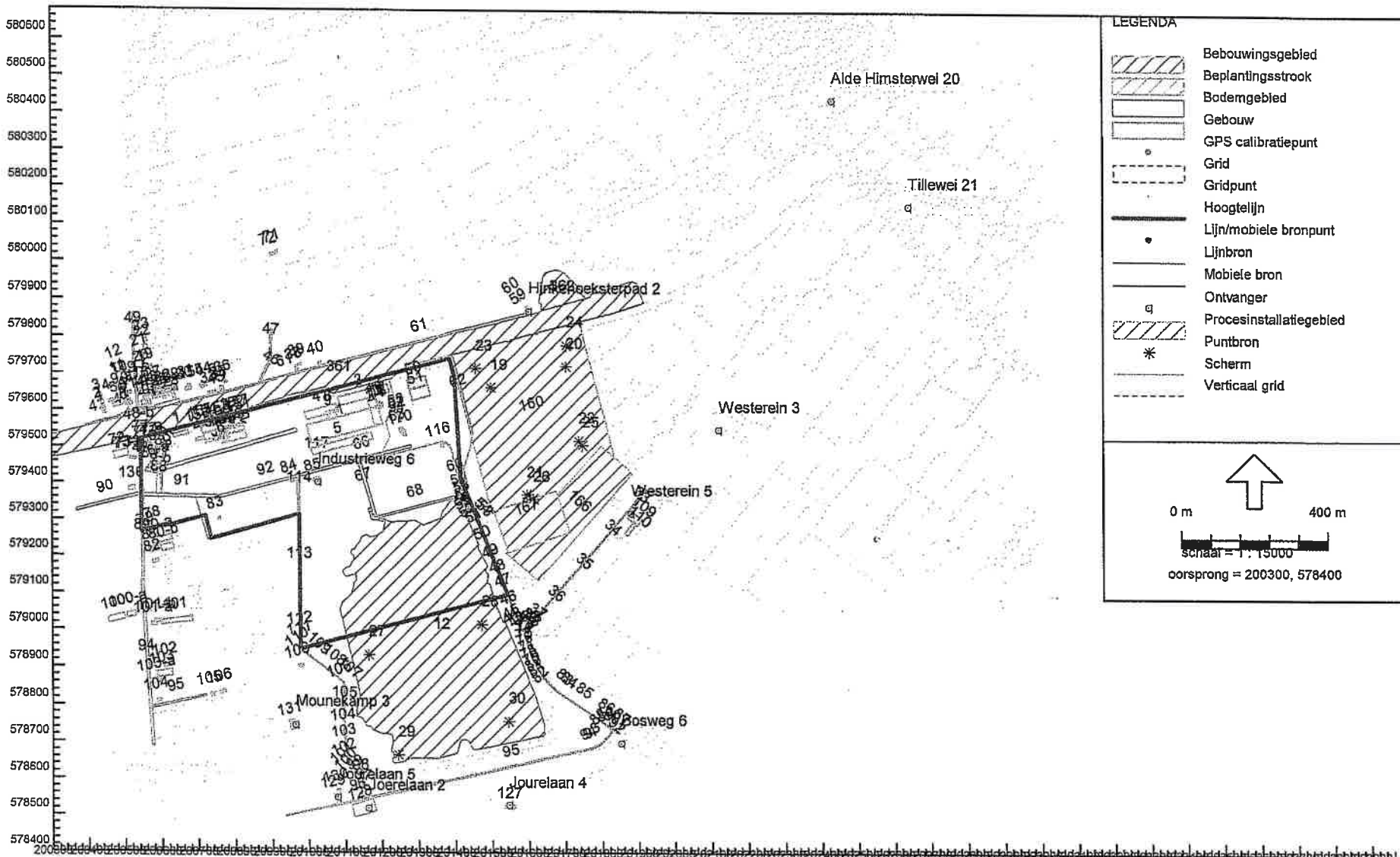
Industrielaai - IL, Schuilenburg - Zonebeheer - Heechsan Zandwinlocatie Schuilenburg niet gez [D:\d06352\Mijn Documenten\Geonoise tijdelijk\VL\OW\Kille_Schuilenburg GNProj_2006-04-03] , Geonoise V5.13
