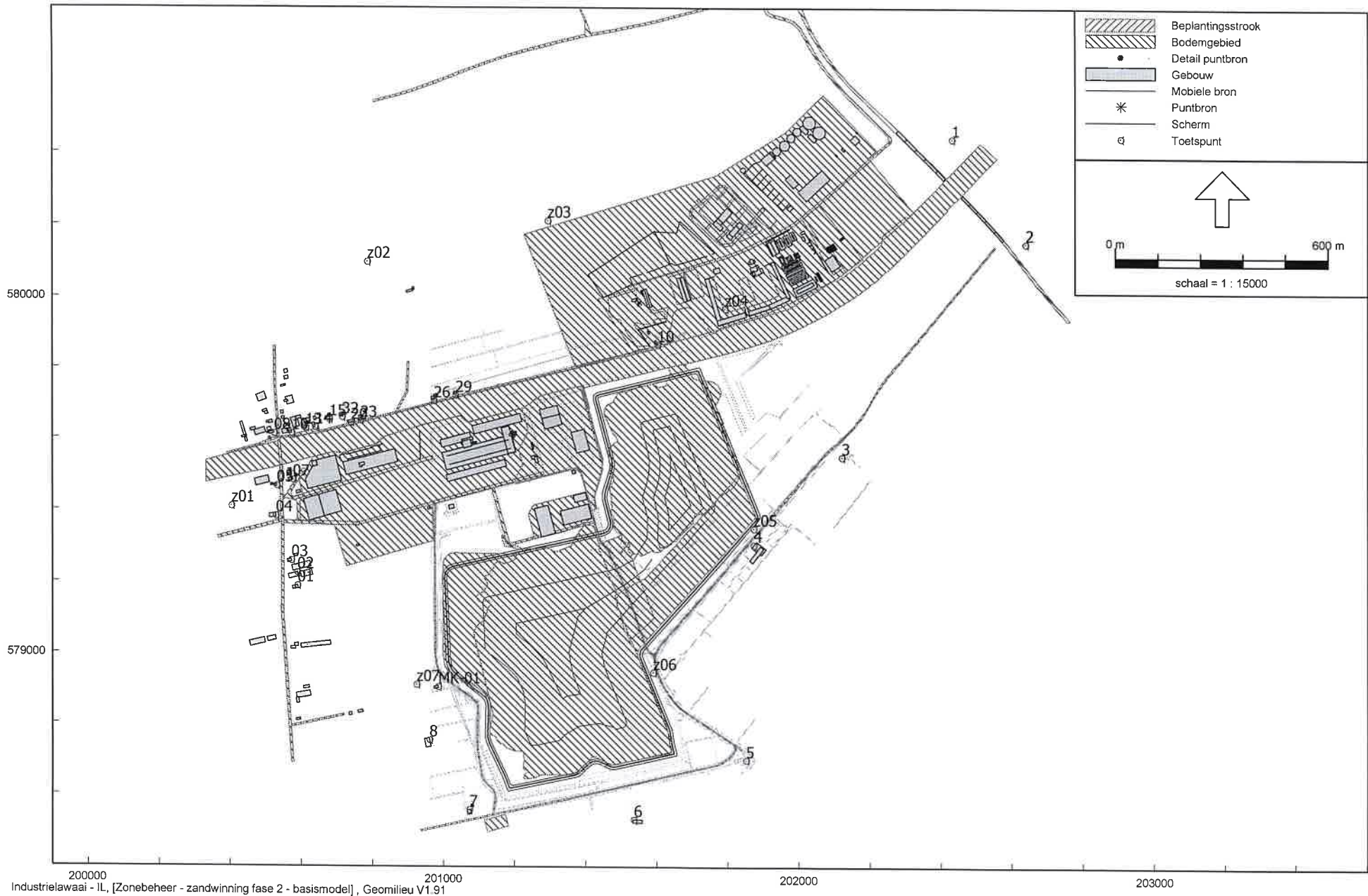
Overzicht van het rekenmodel (exclusief geluidsbronnen) Incl. dxf-ondergrond
